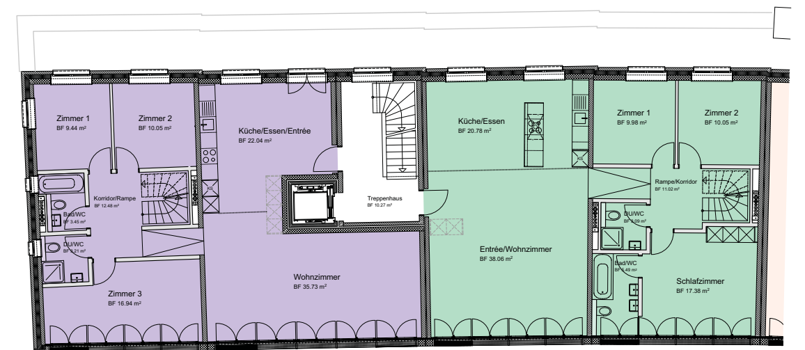
3. Obergeschoss Mst. 1:200
