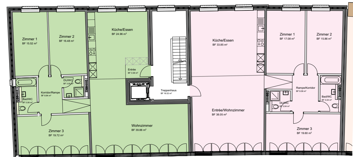
1. Obergeschoss Mst. 1:200
