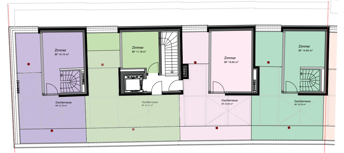
Dachgeschoss Mst. 1:200
