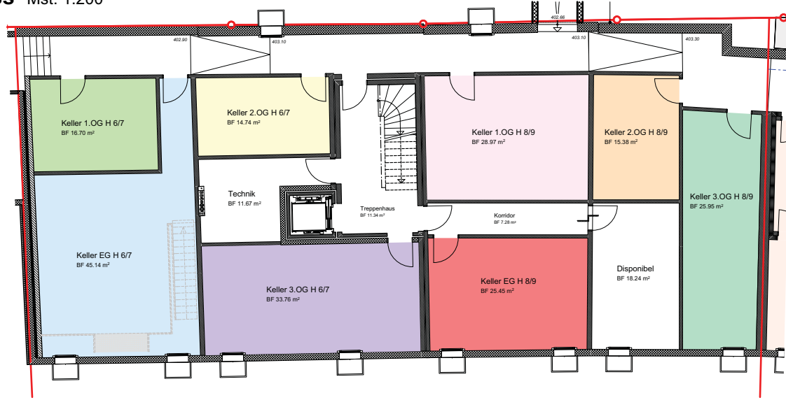
Untergeschoss Mst. 1:200
