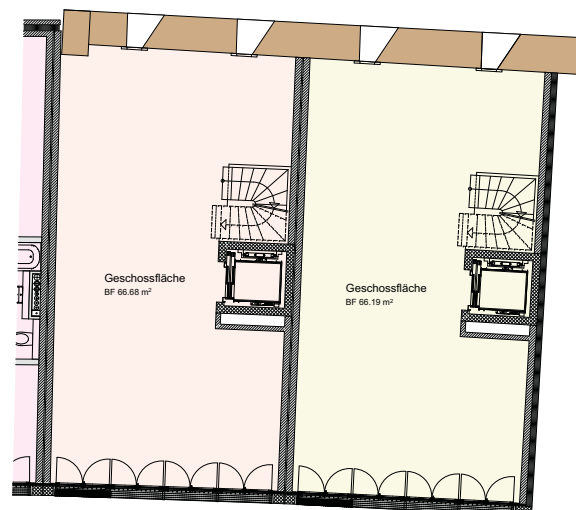
1. Obergeschoss Mst. 1:200
